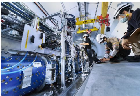
(左図) FASER 検出器の試運転の様子。右側がシリコン検出器の責任者を務める音野助教(九州大学)。
